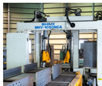
●H形鋼開先加工機 サイズ1000×500
